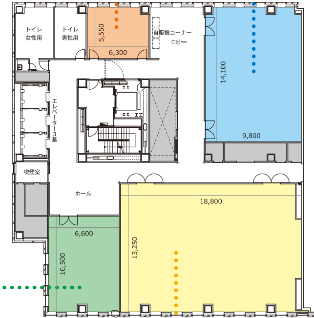
8階平面図
